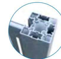
Poteau 90 x 90 mm. Insertion des panneaux en ligne droite ou à 90°.
