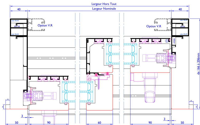
coupe horizontale
