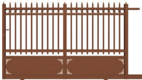
Coulissant : barreaux Ø 20 mm, tôle ép. 3 mm personnalisée motifs d'angle Mélodie et fers de lance pointe Coloris : tanami
