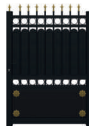
Portillon : barreaux Ø 20 mm, tôle ép. 3 mm, feston ép. 2 mm, fers de lance fleur de lys et marguerites Coloris : noir foncé RAL 9005, bi-coloration sur les ornements
