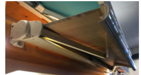
Bras testés à 20 000 cycles dotés d'une articulation à double câble gainé.
