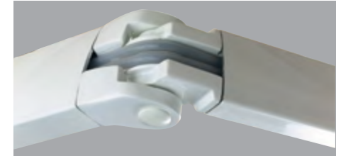
Bras testés à 20 000 cycles dotés d'une articulation à double câble gainé.
