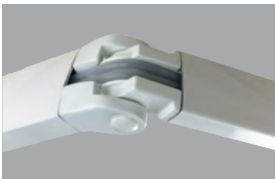
Modèle Grenat Jade Bras à double câbles gainés, testés à 20 000 cycles.
