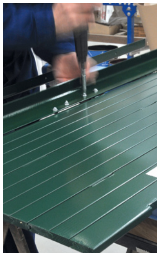
PRÉMONTAGE EN ATELIER des tapées cornières et accessoires
