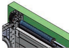
Torsion Avant avec sécurité parachute
