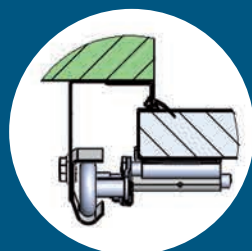
Joint détaché à doubles lèvres périphérique
