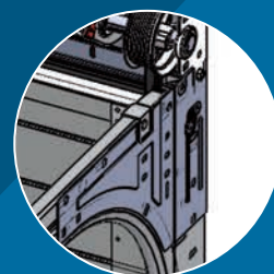
Renfort d'angle sur courbe de renvoi
