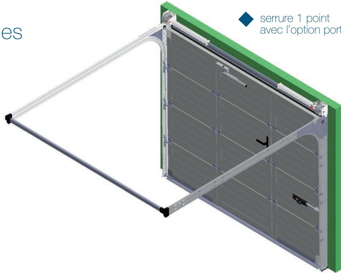
Vue extérieure
