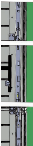
Serrure 3 points inox (5 points d'encrage)
