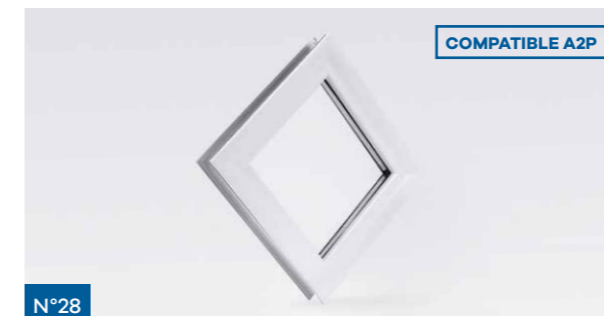
N°28 Entourage : 424 x 424 mm Clair de vitrage : 282 x 282 mm
