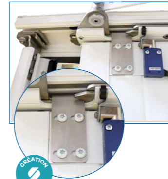
VERROUILLAGE MÉCANIQUE DU PORTILLON DÈS QUE LA PORTE DE GARAGE S'OUVRE
